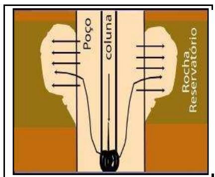
Figura 2.5.1: Esquematização da invasão de filtrado do poço para a rocha reservatório
